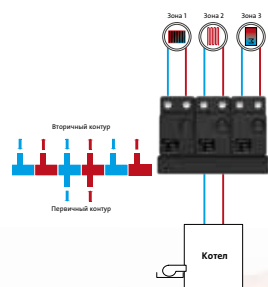
Пример монтажа насосных групп HEATMIX с коллектором без гидроразделителя
